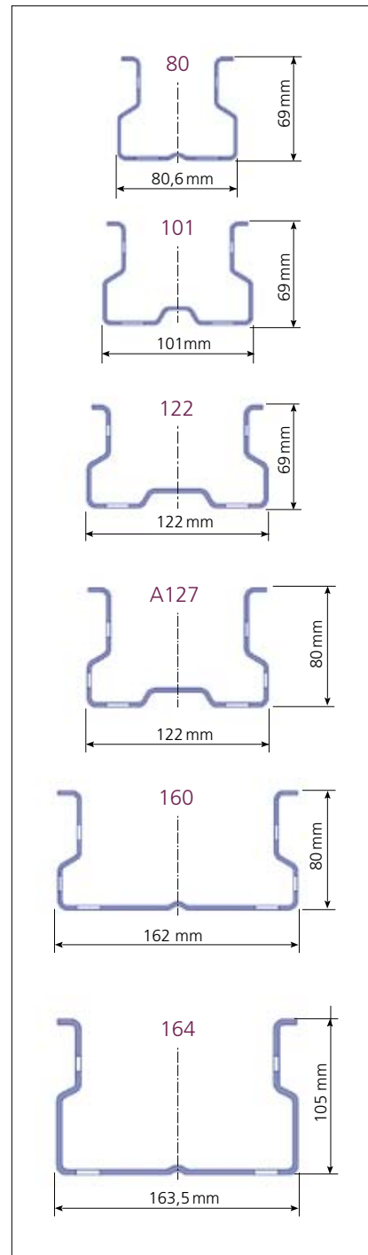
Figura 8. Puntales empleados.
